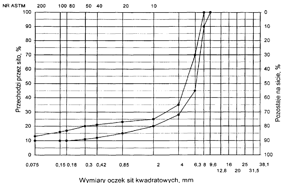
uziarnienia mieszanki mineralnej SMA od 0 do 8 mm do warstwy ścieralnej nawierzchni drogi o obciążeniu ruchem od KR3 do KR6
