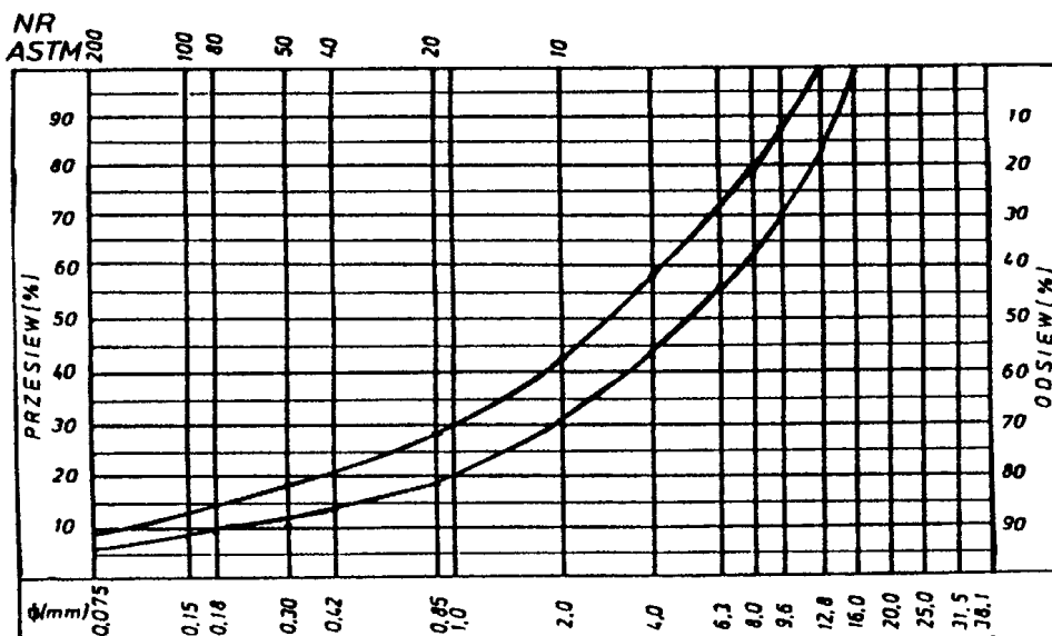
graniczne uziarnienia mieszanki mineralnej 0+16 mm do warstwy ścieralnej z betonu asfaltowego dla KR 3-6
