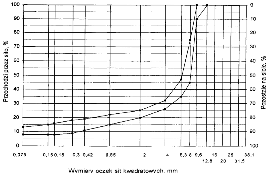
graniczne uziarnienia mieszanki mineralnej SMA od 0 do 9,6 mm do warstwy ścieralnej nawierzchni drogi o obciążeniu ruchem od KR3 do KR6
