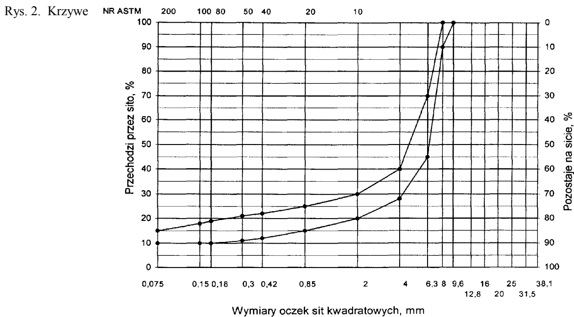
Rys. 2. Krzywe graniczne uziarnienia mieszanki mineralnej SMA od 0 do 8 mm do warstwy ścieralnej nawierzchni drogi o obciążeniu ruchem KR1 lub KR2
