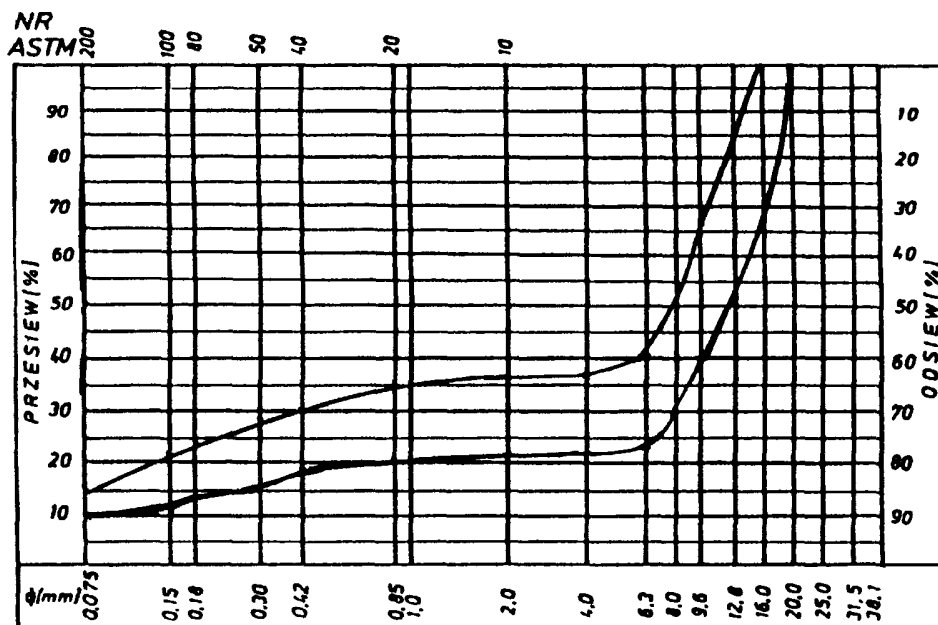
graniczne uziarnienia mieszanki mineralnej 0+20 mm o nieciągłym uziarnieniu do warstwy ścieralnej z betonu asfaltowego dla KR 3-6
