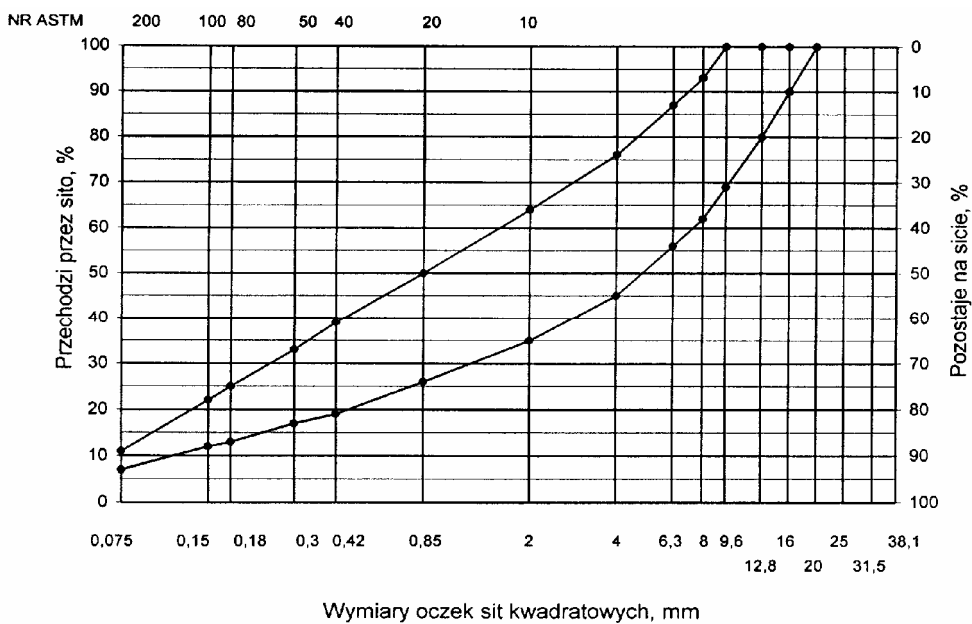
Wymiary oczek sit kwadratowych, mm Rys. 2. Krzywe graniczne uziarnienia mieszanki mineralnej BA od 0 do 16mm, od 0 do 12,8 mm do warstwy ścieralnej nawierzchni drogi o obciążeniu ruchem KR1 lub KR2
